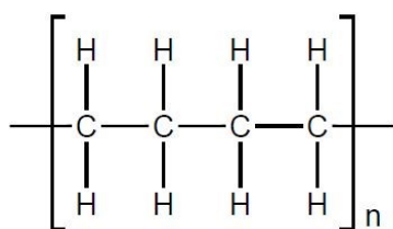
Polythene (poly(ethene))
