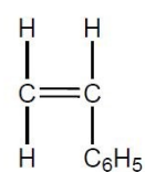
Styrene
