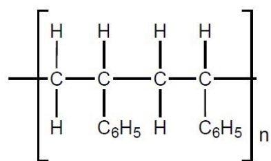
Polystyrene
