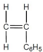
Styrene
